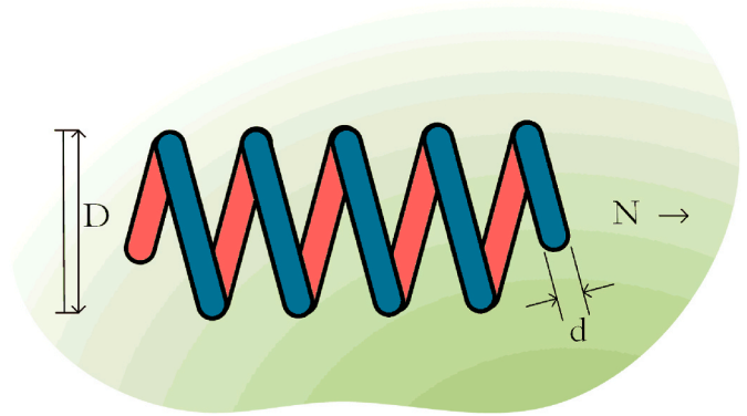
Fig. 12. TSD problem.
