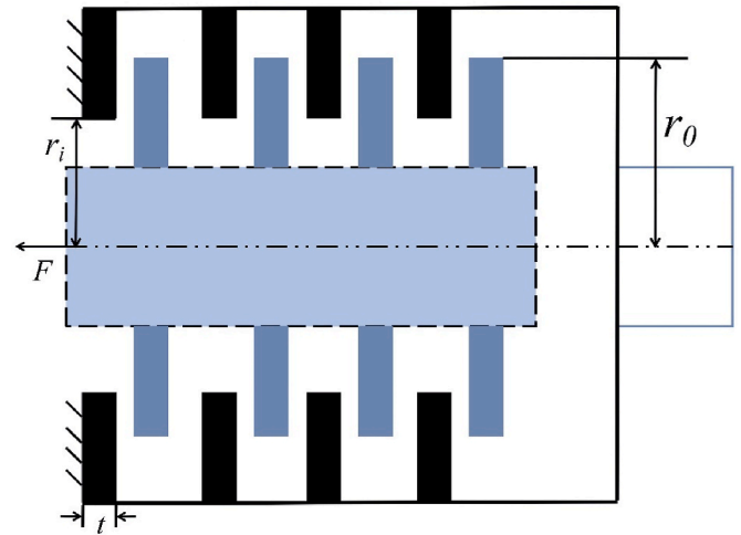
Fig. 14. MDCBD problem.
